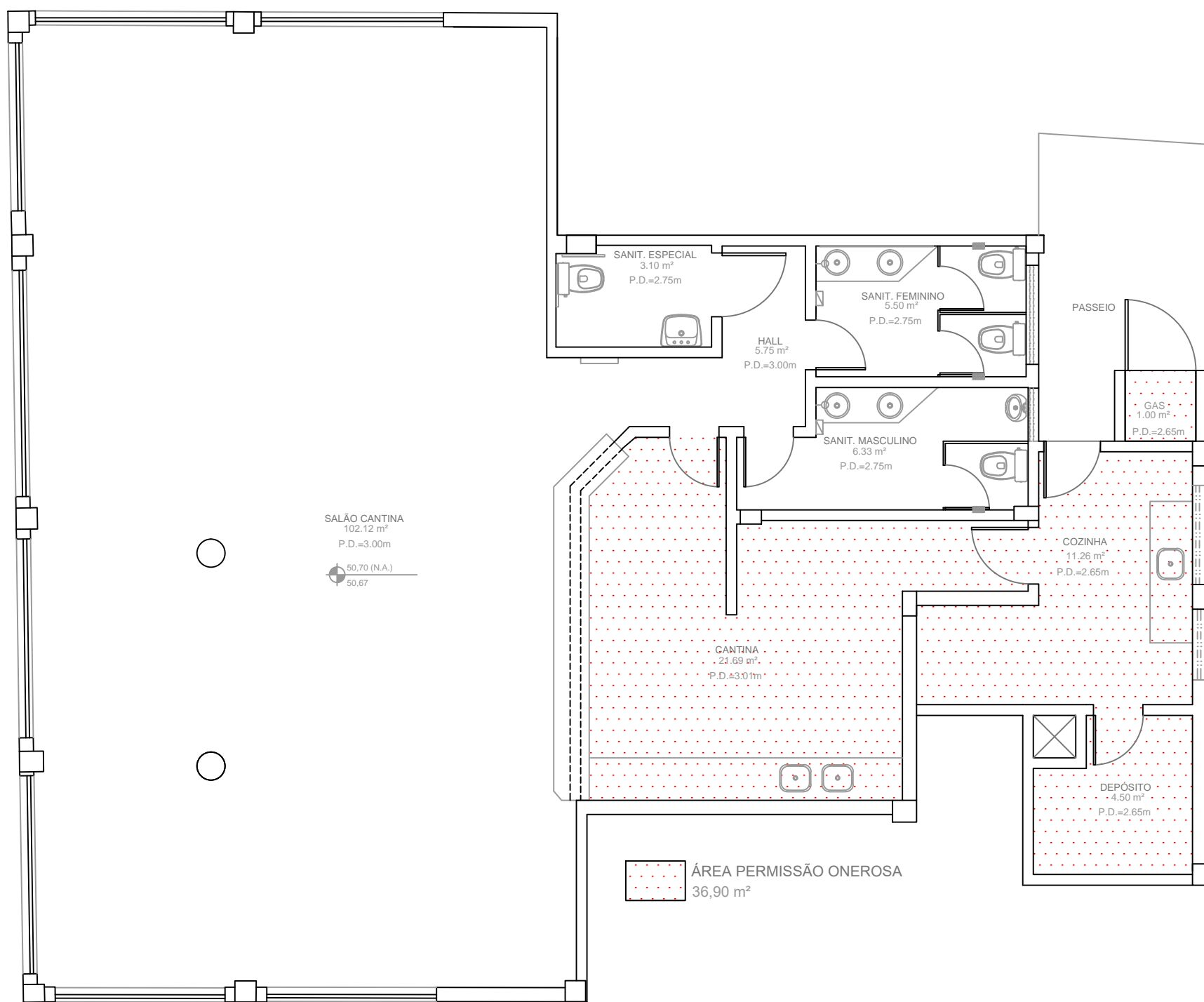
01 PLANTA BAIXA - TÉRREO 1/150
